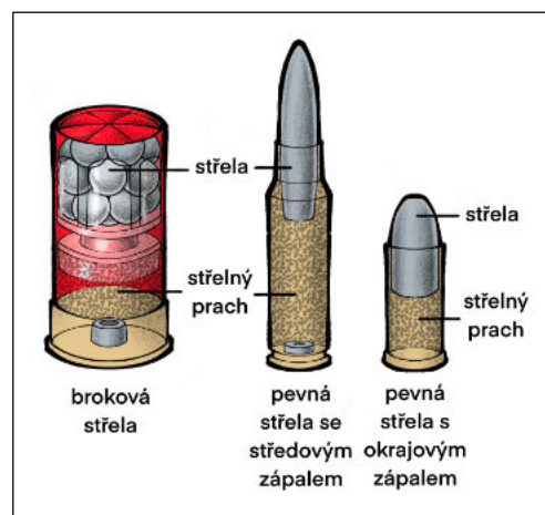
Stavba rozdílných typů nábojů (kresba David Říha).
