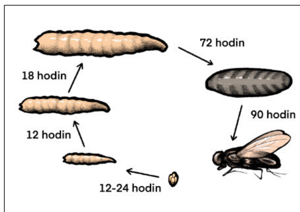
Časové schéma vývoje různých stadií mouchy bzučivky na zvířecím kadáveru při 21°C (kresba David Říha).
